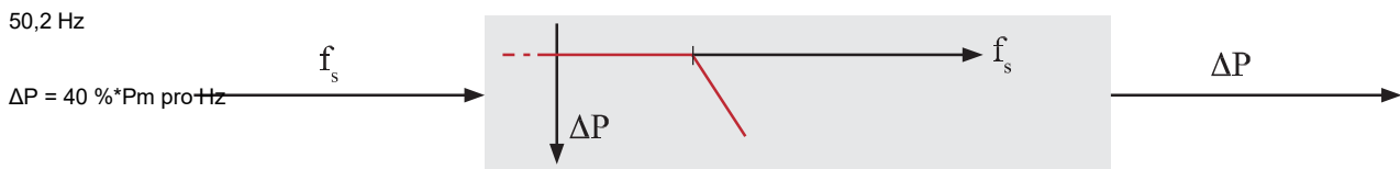
Obrázok 1 - Zníženie činného výkonu v závislosti od frekvencie siete
